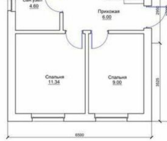
Разбивочный план 2-го этажа
