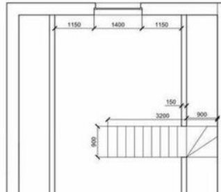
Разбивочный план 2-го этажа
